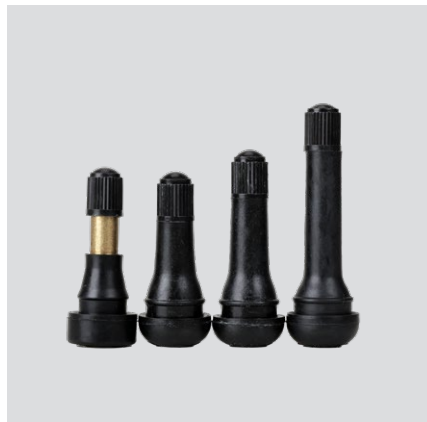
ट्यूबलेस टायर वाल्व TR413, TR414, TR418, TR600HP सभी ट्यूबलेस रिम्स के लिए R2749
